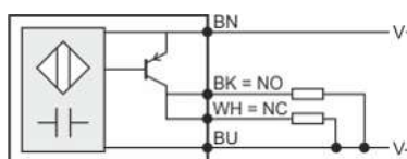
(i)DOL 27 PNP
