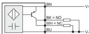
(i)DOL 26 PNP
