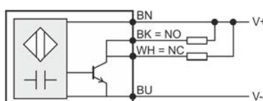
(i)DOL 26 NPN
